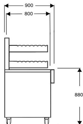
M25C2 2 Tier Charcoal Rotisserie
